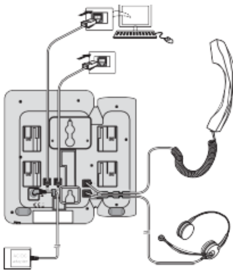
Fig. 1: conexión serie 1000i
